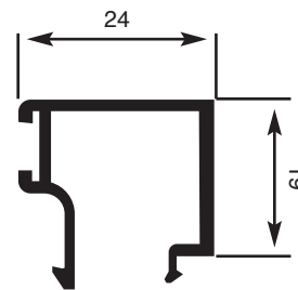
AH-9007 Junquillo para Hoja A-03863
